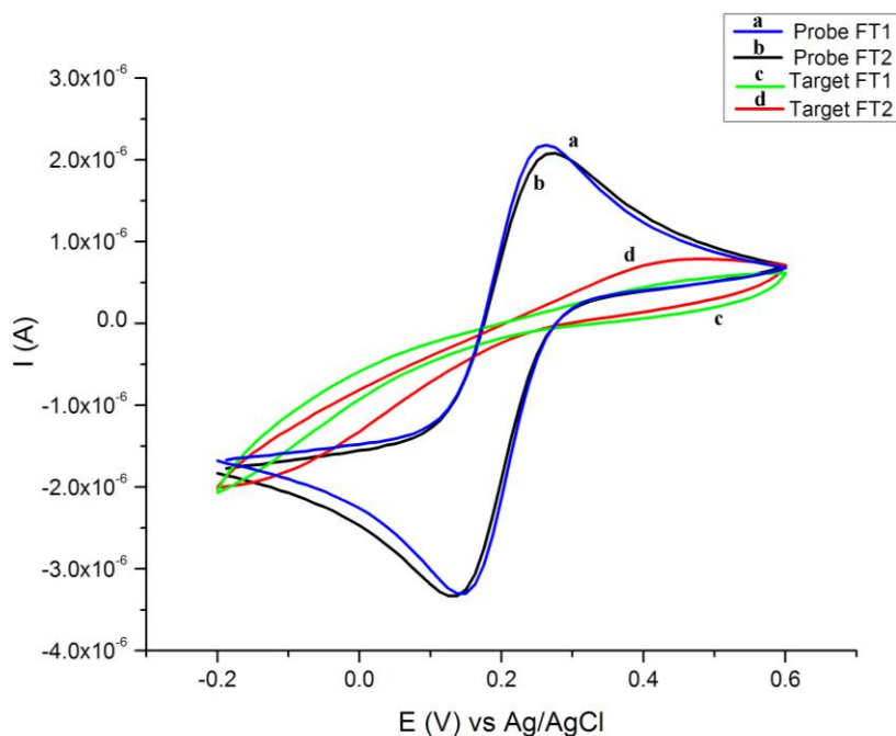
Hình 5. Hiệu quả giải hấp lớp màng SAM. (A), (B) cường độ dòng khi gắn probe lần 1 và lần 2; (C), (D) cường độ dòng khi lại với mục tiêu lần 1 và lần 2.
