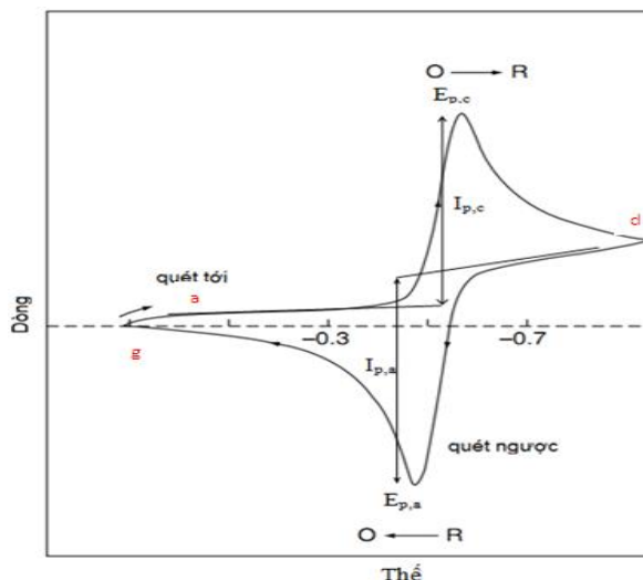
Hình 2. Đặc trưng CV của hệ oxy hóa khử thuận nghịch O + ne^- \rightleftharpoons R .
