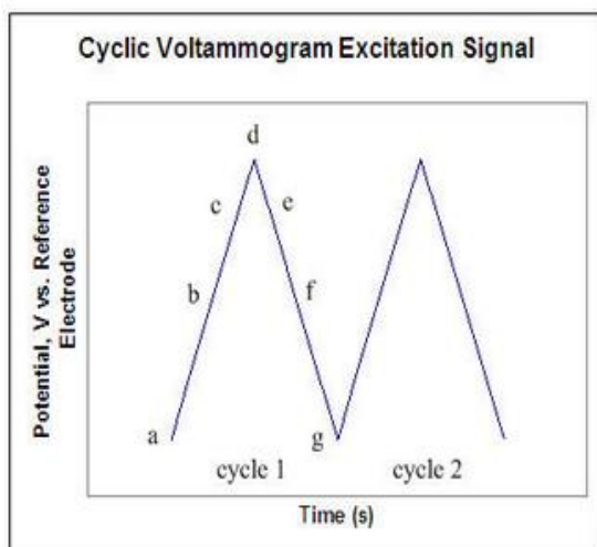
Hình 1. Biểu diễn quá trình khử xảy ra khi quét theo chiều âm từ (a) đến (d) và quá trình oxy hóa xảy ra khi quét theo chiều dương từ (d) đến (g). Quét thế vòng tuần hoàn thu được kết quả về dòng điện ở điện cực làm việc trong quá trình quét thế.
