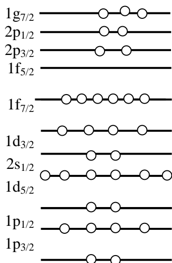
Hình 11. Mức kích thích thứ chín.
