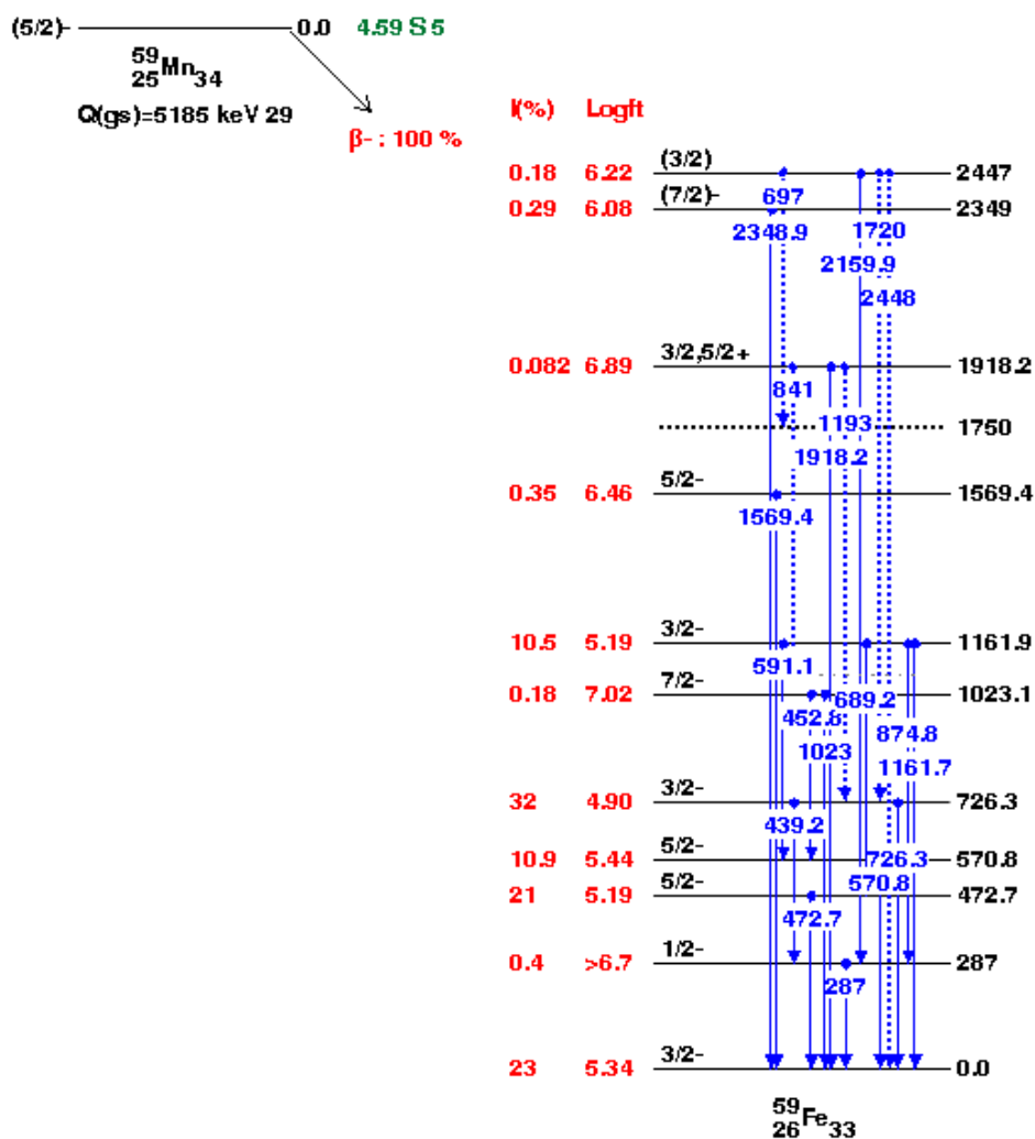
Hình 13. Các mức kích thích của ^{59}\text{Fe} đo được từ phát beta của đồng vị ^{59}\text{Mn} [8].
