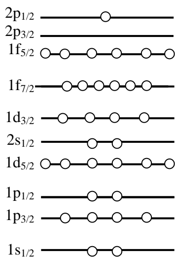
Hình 3. Mức kích thích thứ nhất.
