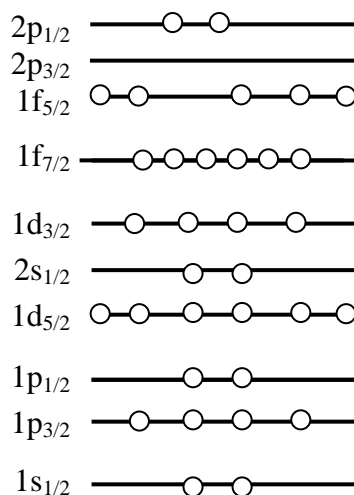
Hình 4. Mức kích thích thứ hai.
