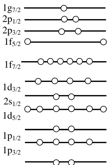
Hình 7. Mức kích thích thứ năm.
