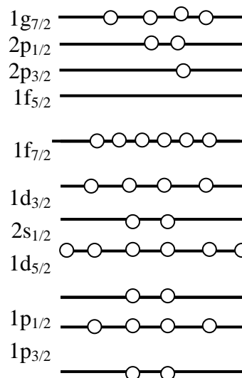
Hình 12. Mức kích thích thứ mười.
