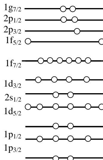
Hình 8. Mức kích thích thứ sáu.
