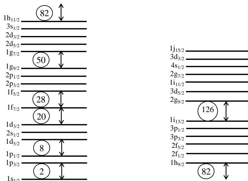
Hình 1. Sơ đồ các mức nucleon trong hạt nhân theo mẫu lớp.
