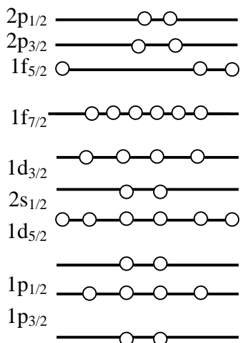
Hình 5. Mức kích thích thứ ba.
