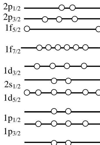
Hình 6. Mức kích thích thứ tư.
