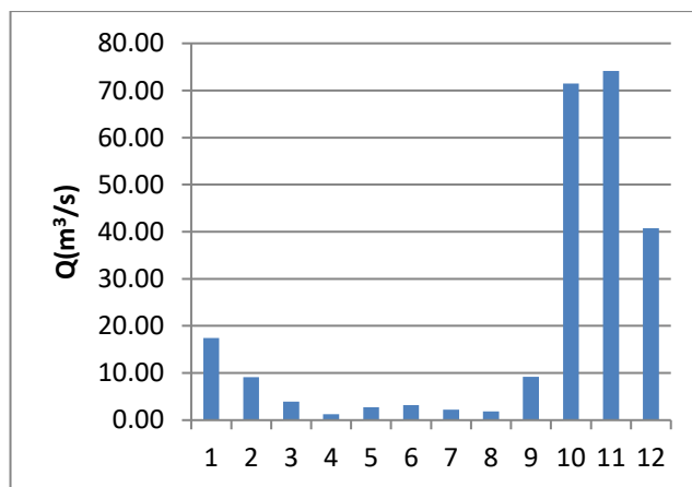
Hình 6. Biểu đồ lưu lượng trung bình tháng sông Hà Thanh
