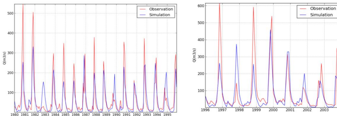
Hình 4. Kết quả hiệu chỉnh (trái), kiểm định (phải) với bước thời gian tháng
