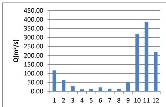
Hình 5. Biểu đồ lưu lượng trung bình tháng sông Kôn
