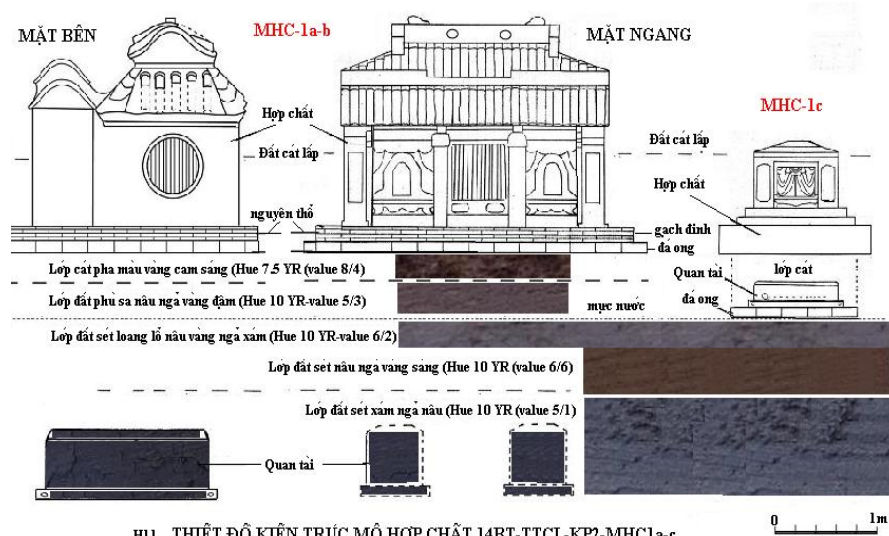
H11. THIẾT ĐỒ KIẾN TRÚC MỘ HỘP CHẮT 14BT-TTCL-KP2-MHC1a-c
