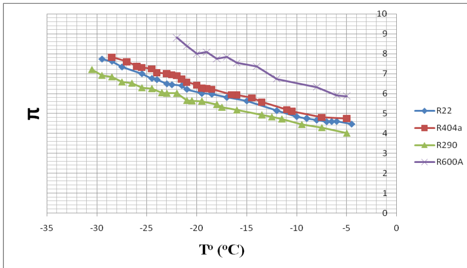
Hình 2. Mối quan hệ giữa nhiệt độ sôi và tỷ số nén tại nhiệt độ môi trường 29°C.
