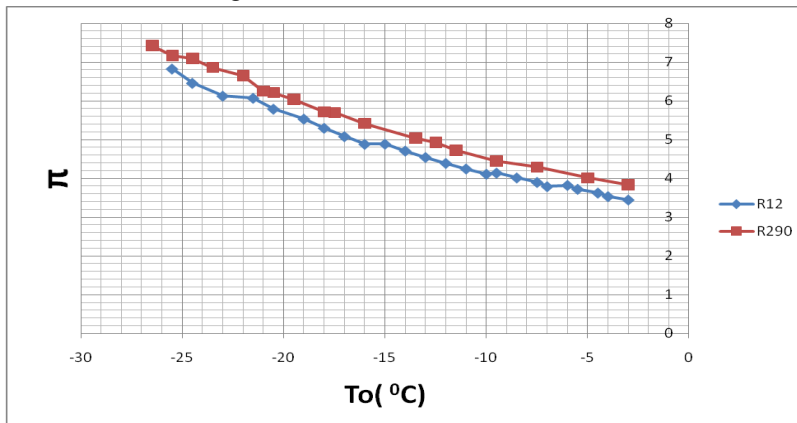
Hình 5. Biến thiên tỷ số nén và nhiệt độ bay hơi tại nhiệt độ môi trường 29°C
