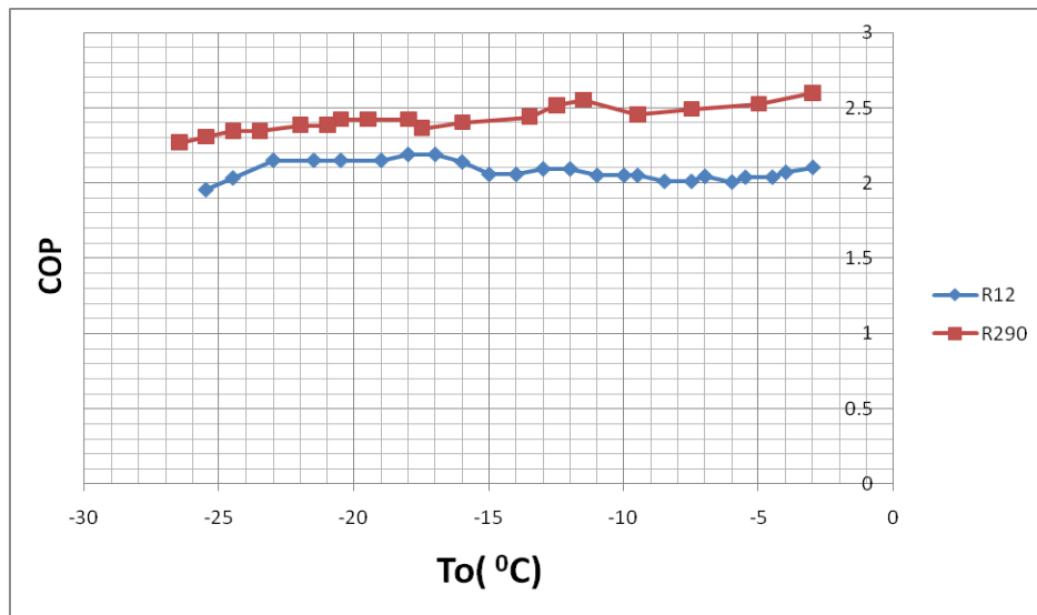
Hình 7. Mối quan hệ giữa COP và nhiệt độ bay hơi
