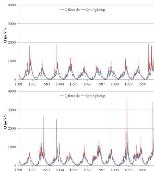
Hình 6. Đường so sánh quá trình lưu lượng thực đo và tính toán tại trạm Bản Đôn; giai đoạn hiệu chỉnh (bên trên) và giai đoạn kiểm định (bên dưới)
