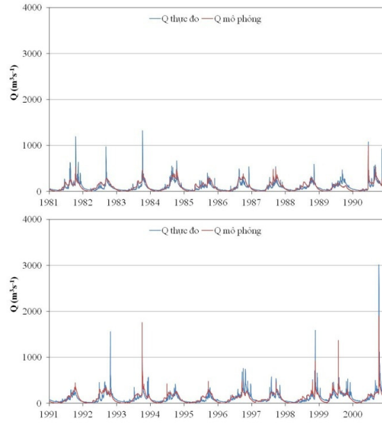
Hình 4. Đường so sánh quá trình lưu lượng thực đo và tính toán tại trạm Đức Xuyên; giai đoạn hiệu chỉnh (bên trên) và giai đoạn kiểm định (bên dưới)
