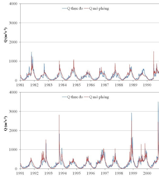
Hình 5. Đường so sánh quá trình lưu lượng thực đo và tính toán tại trạm Cầu 14; giai đoạn hiệu chỉnh (bên trên) và giai đoạn kiểm định (bên dưới)
