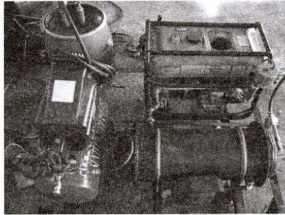
Hình 5. Mô hình thí nghiệm động cơ biogas.
