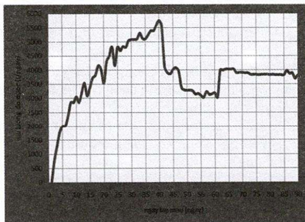
Hình 1. Biểu đồ sinh khí biogas của một mê ủ ( 5 \text{ m}^3 ) lấy khí trong vòng 3 tháng.
