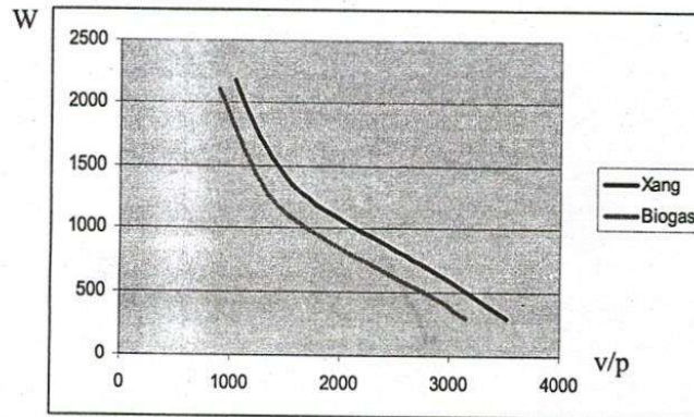
Hình 6. Đồ thị so sánh công suất máy điện khi động cơ dùng nhiên liệu xăng và biogas
