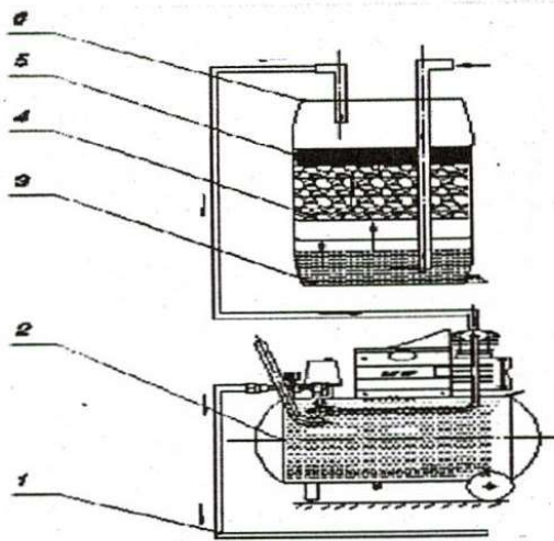
Hình 2. Sơ đồ nguyên lý lọc khí Biogas
