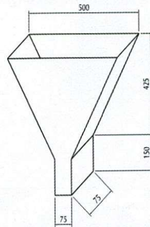
Hình 5. V-funnel
