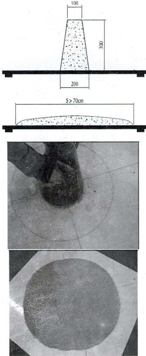
Hình 5. Thí nghiệm độ chảy
