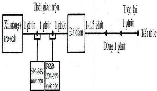
Hình 7. Quy trình trộn bê tông
