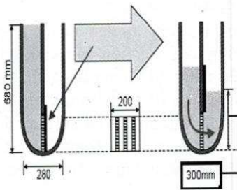
Hình 3. U-flow test
