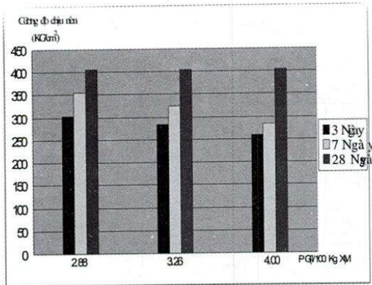
Hình 2. Ảnh hưởng của hàm lượng phụ gia dẻo đến sự phát triển cường độ của bê tông tự lên
