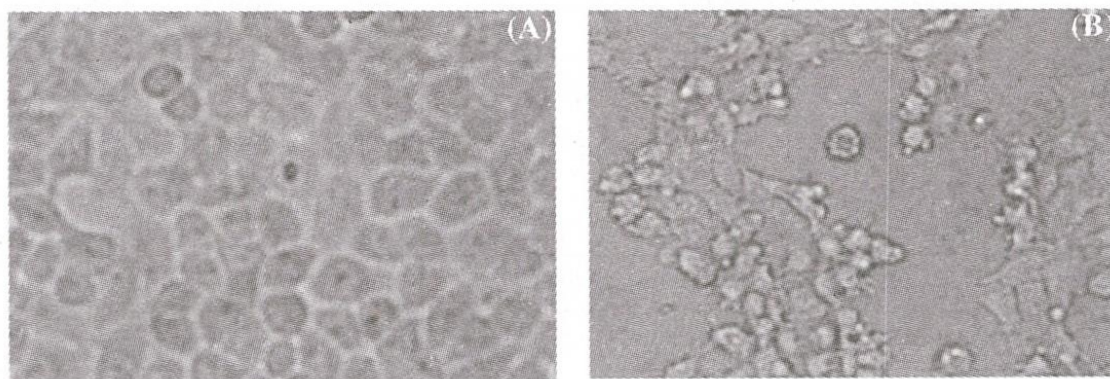
Hình 1: Tế bào HeLa được quan sát dưới kính hiển vi soi ngược (400X).
