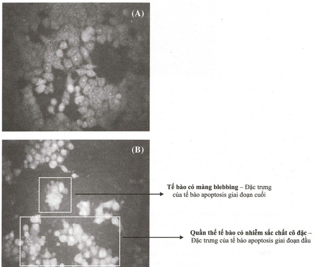
Hình 2. Tế bào HeLa được quan sát dưới kính hiển vi huỳnh quang (400x). (A). Tế bào không xử lý với thuốc (B). Tế bào được xử lý với cao chiết PEE nồng độ 1 \mu\text{g/ml} trong 24 giờ
