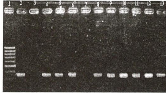
Hình 4. Kết quả điện di sản phẩm PCR
