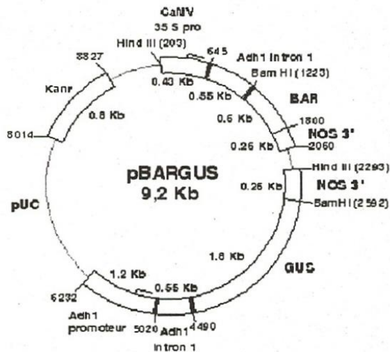
Hình 1: Plasmid pBAR-GUS
