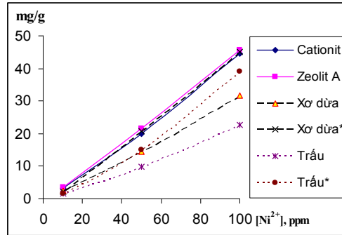
Hình 3. Dung lượng xử lý Nickel
