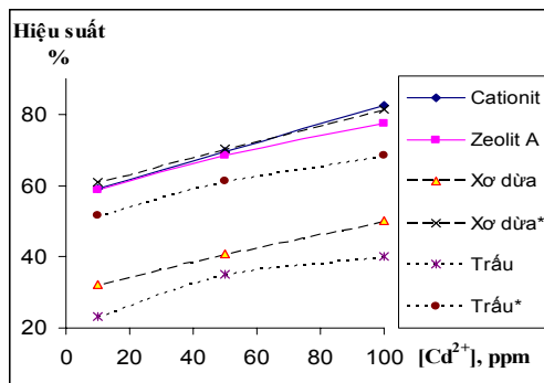
Hình 4. Hiệu suất xử lý Cadmium
