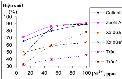
Hình 2. Hiệu suất xử lý Nickel
