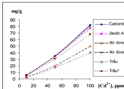
Hình 5. Dung lượng xử lý Cadmium
