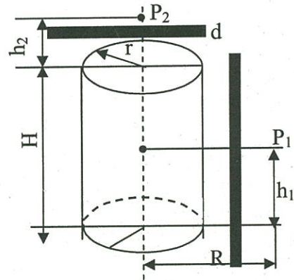
Hình 2. Nguồn gamma dạng mặt trụ có tấm che bề dày d
