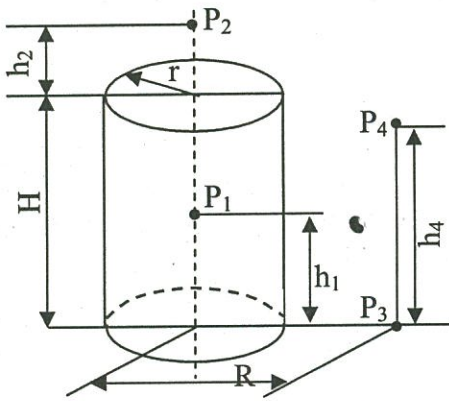
Hình 1. Nguồn gamma dạng mặt trụ không che chắn
