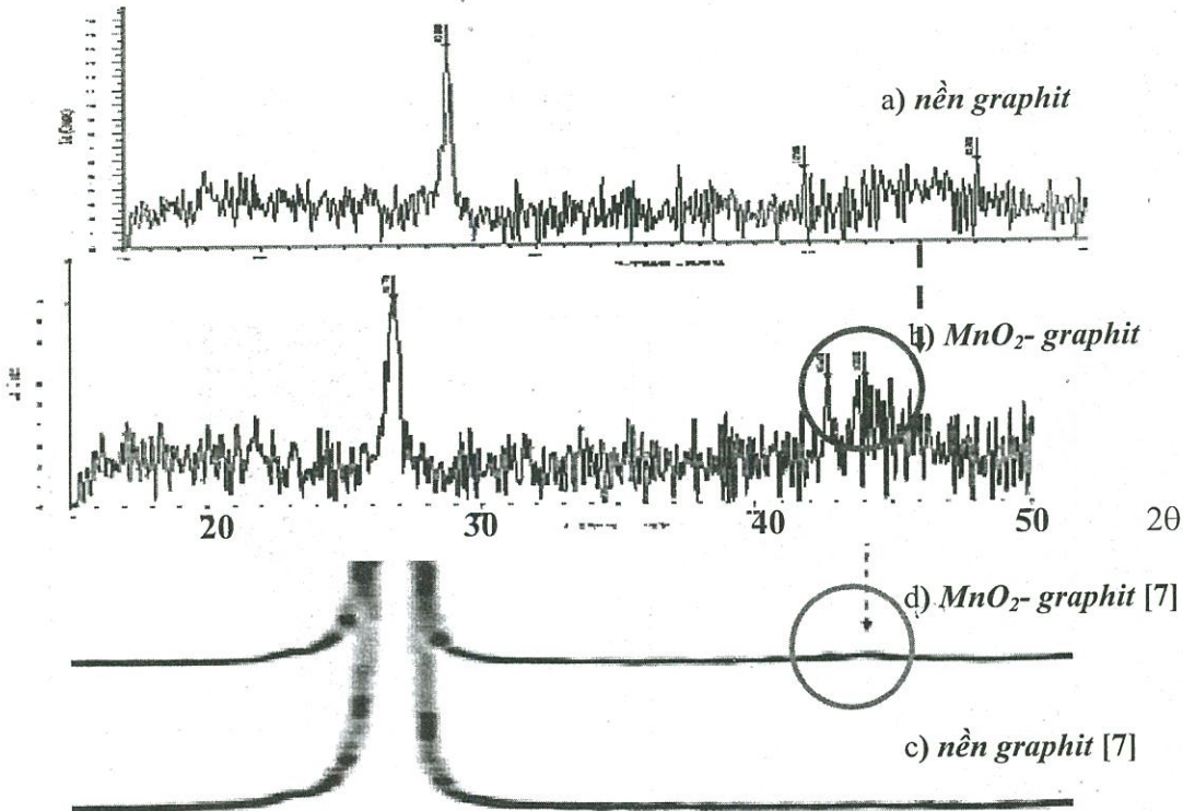
Hình 4: Phổ XRD của nền graphit (a) và MnO_2 kết tủa (b) ở mật độ dòng 0,20 \text{ mA/cm}^2 ; (c, d) là phổ XRD trích dẫn từ công trình [8].
