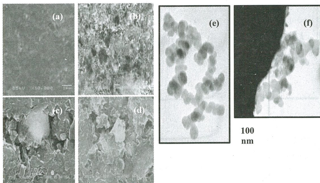
Hình 3: Ảnh SEM của MnO 2 tạo thành trên nền graphit với các mật độ dòng khác nhau: a) 0,2; b) 0,4; c) 0,6; d) 1,0 mA/cm 2 . Ảnh TEM của mẫu MnO 2 kết tủa ở i = 0,2 mA/cm 2 : e) bề mặt và f) mặt cắt ngang.
