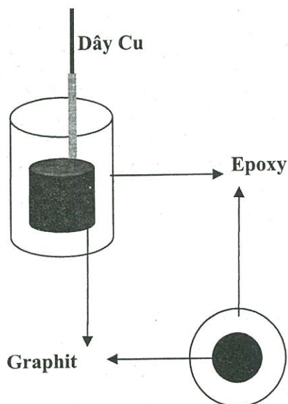
Hình 1: Điện cực graphit (trên) và mặt cắt ngang (dưới).
