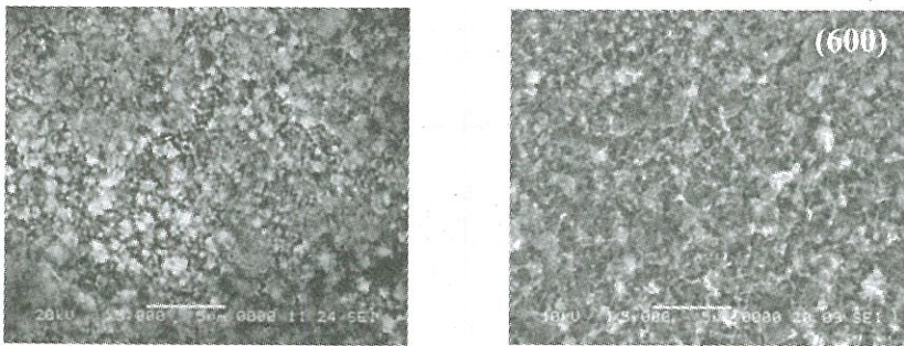
Hình 8: Ảnh SEM của điện cực MnO_2/C_{sl} trước (1) và sau 600 chu kỳ quét thế (600). Tốc độ 50 mV/s, KCl 2 M, 25°C.
