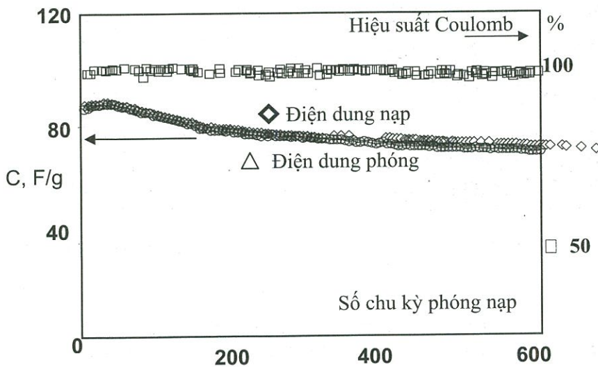
Hình 6: Biến thiên điện dung và hiệu suất coulomb của điện cực MnO 2 /Csl theo số vòng quét thế.
