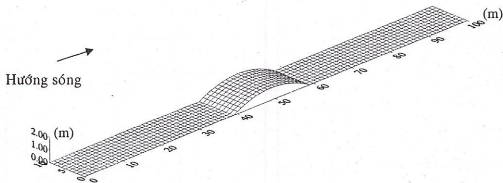
Hình 2 : Vị trí ban đầu mô cát
