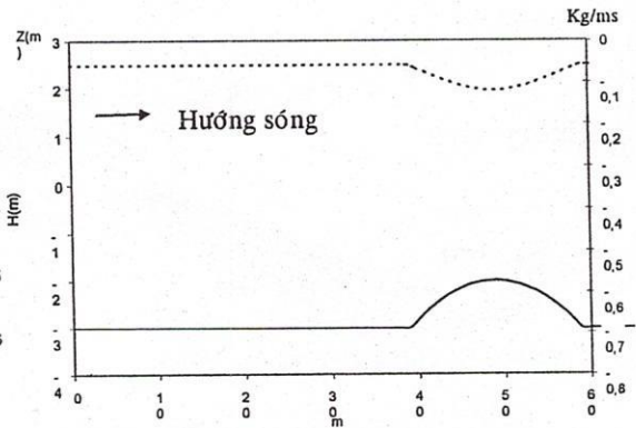
Hình 4. Profile của mô cát (—) và sức tải cát
