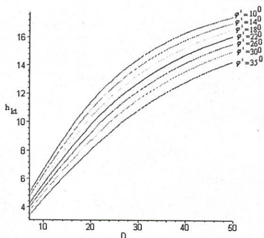
H.4 - Biểu đồ quan hệ giữa h_{kt} và D khi \varphi' thay (theo số liệu bảng 2)
