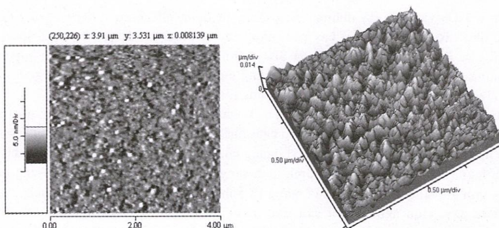
Hình 1a. \text{TiO}_2\text{-SiO}_2 (0% \text{SiO}_2 ) : Rms Rough: 6.481 (nm);
