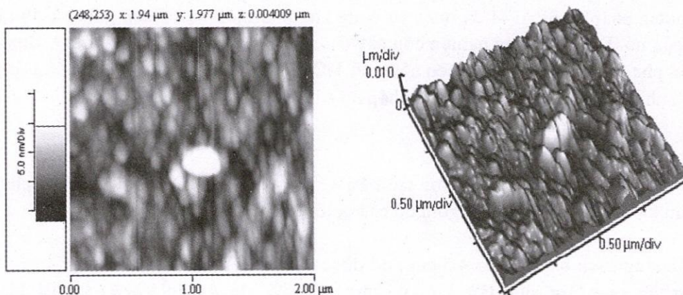
Hình 1a. \text{TiO}_2\text{-SiO}_2 (0% \text{SiO}_2 ) : Rms Rough: 6.481 (nm);
