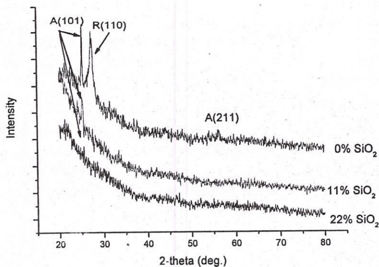
Hình 5. Phổ nhiễu xạ tia X của các màng có tỉ lệ SiO 2 khác nhau được nung ở nhiệt độ 600°C trong 3h.
