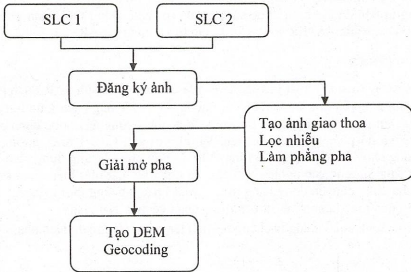
Hình 4. Quy trình xử lý kỹ thuật InSAR
