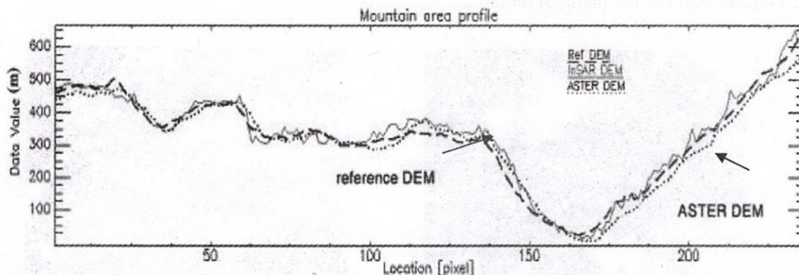
Hình 7b. So sánh cao độ giữa DEM ASTER, DEM INSAR
