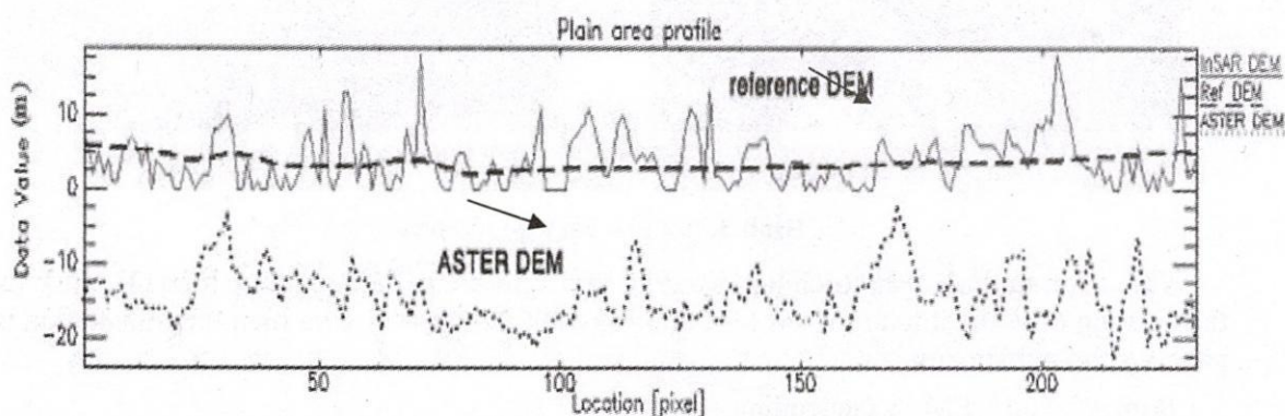
Hình 7a. So sánh cao độ DEM ASTER, DEM INSAR
