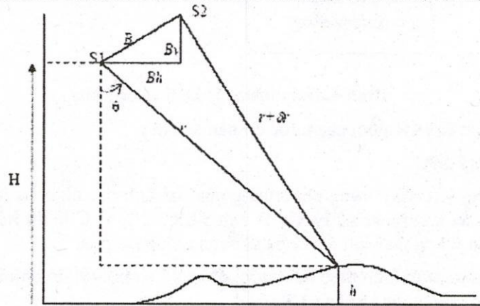
Hình 3. Cấu hình hình học InSAR
