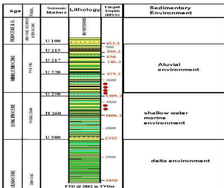
Hình 20. Cột địa tầng của giếng khoan 102 – T – 1X sau phân tích [2]
