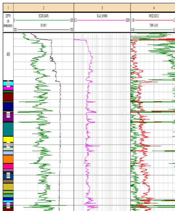
Hình 5. Bảng log cơ sở đánh giá thay đổi của GR
