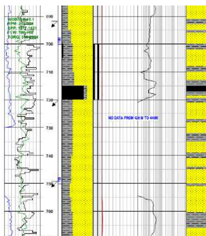
Hình 7. Bảng log độ sâu từ 690 – 770 mMD
