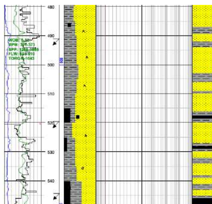
Hình 6. Bảng mudlog mô tả thạch học ở độ sâu 480 – 550 mMD.
