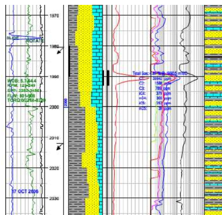
Hình 12. Băng log 1967 – 2037 mMD
