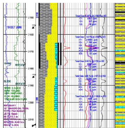
Hình 13. Băng log 2142 – 2216 mMD
