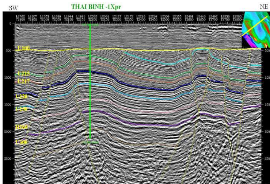
Hình 2. Băng địa chấn tổng hợp phân chia các tập địa chấn - địa tầng [2]
