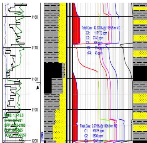
Hình 8. Bảng log độ sâu 1156 – 1203 mMD
