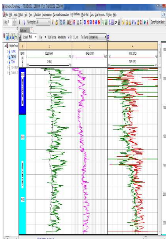
Hình 10. Bảng log cơ sở độ sâu 1000 – 2300 m MD
