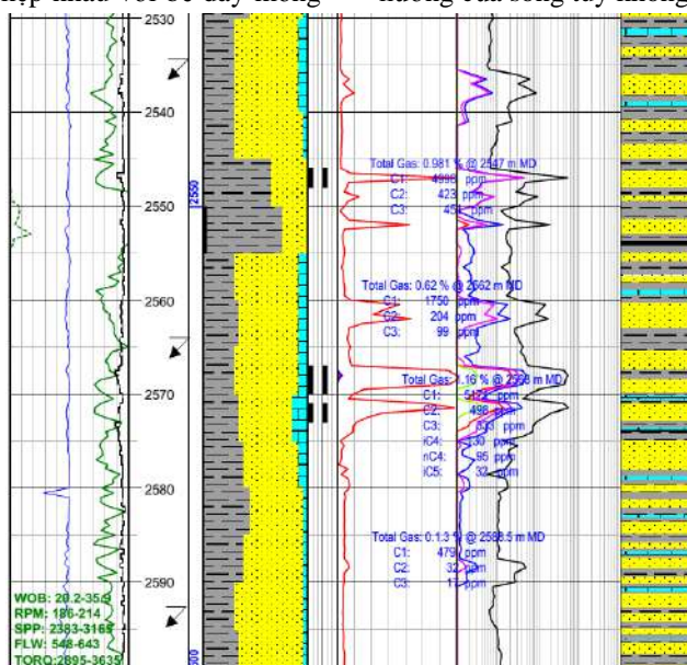
Hình 18. Bảng log từ 2530 – 2594m MD
