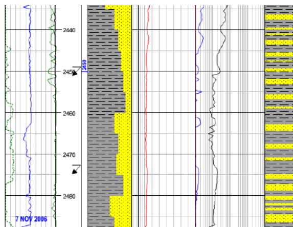
Hình 17. Bảng log từ 2436 – 2487 mMD
